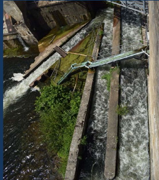
La passe à ralentisseurs à Mauzac barrage
