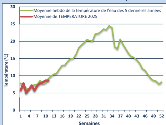
Température moyenne hebdomadaire de la Dordogne
