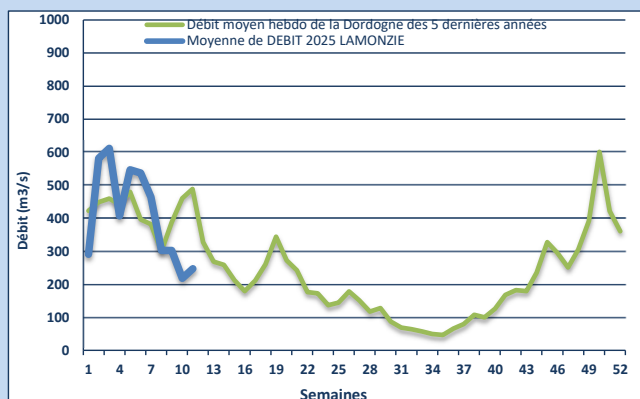
Débit moyen hebdomadaire de la Dordogne
